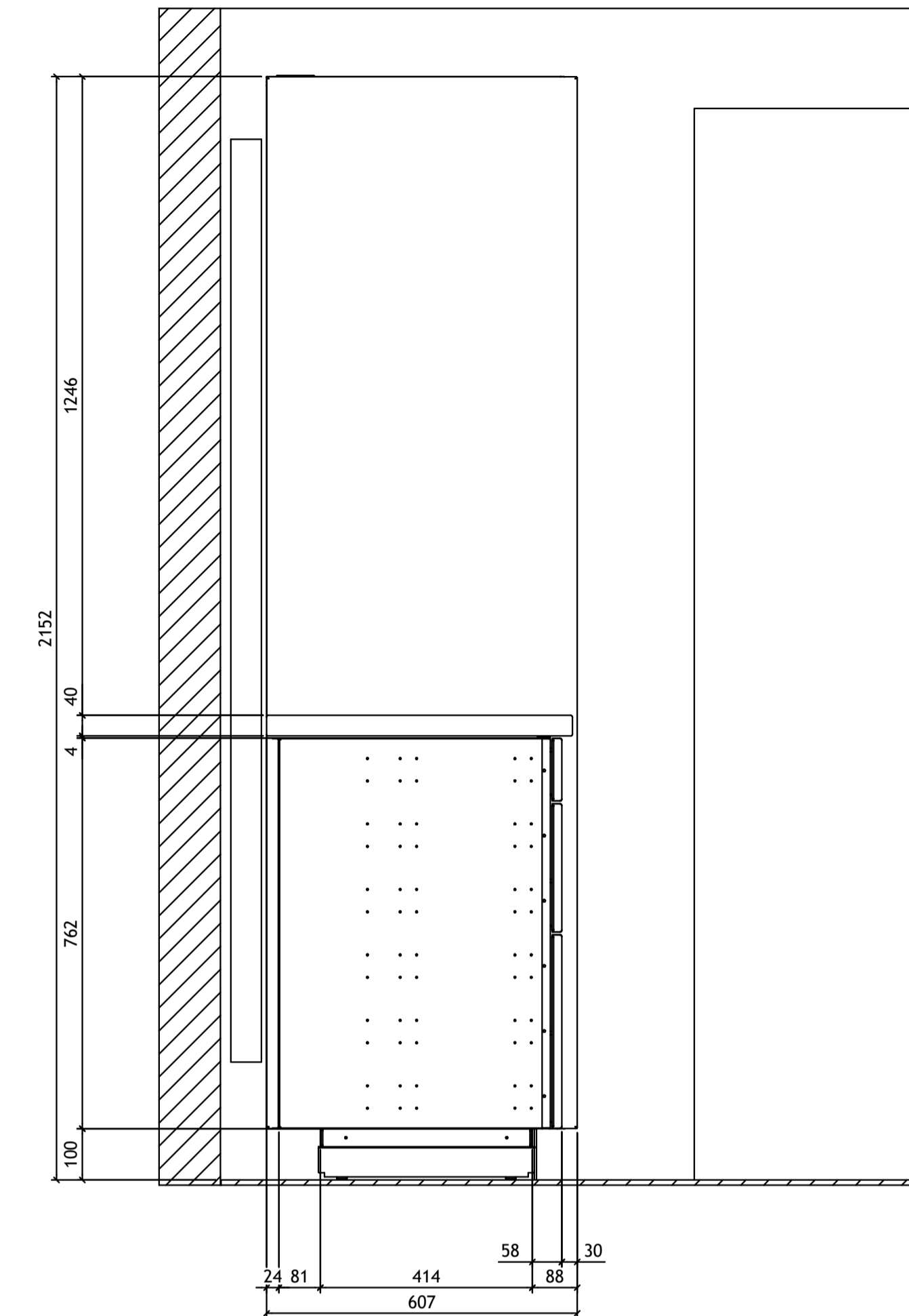
C-C ( 1 : 10 )
