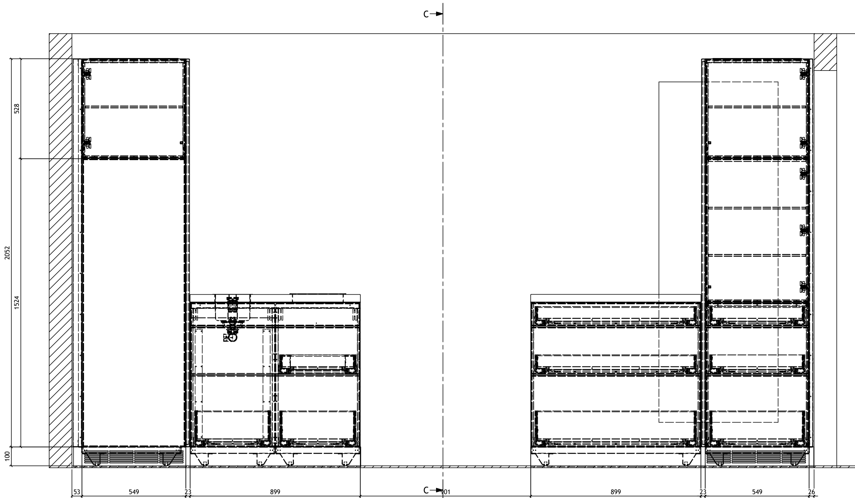
B-B ( 1 : 10 )
