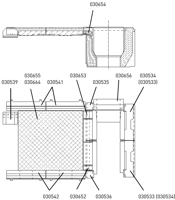
Modell 674 (Abbildung= Feuer rechts / links= spiegelbildlich)
