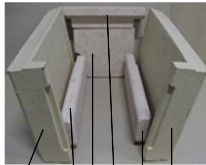
Ausführung mit Heizelement
