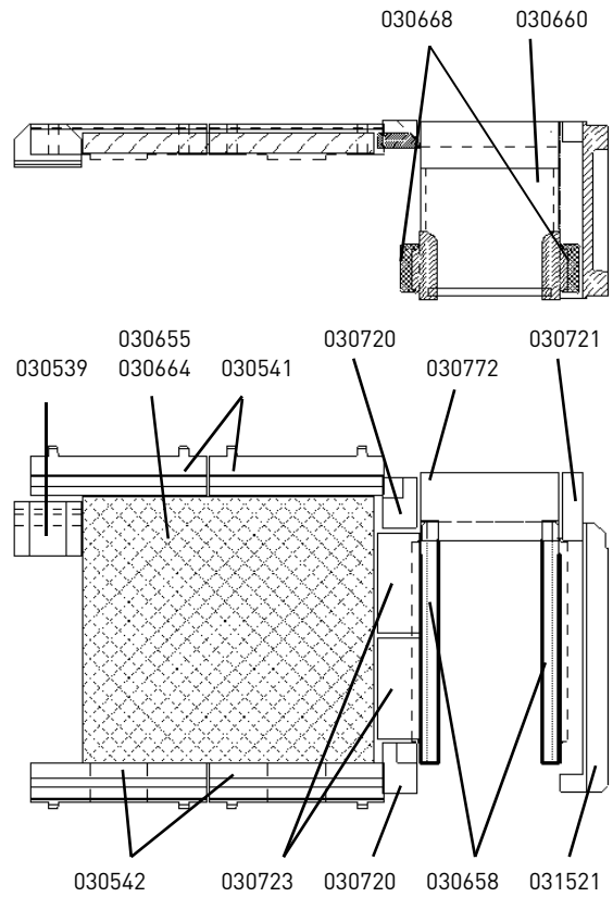
Ausführung mit Heizelement
