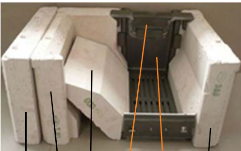
Modell 624 und 634 / Türbandung links (Feuer rechts)
