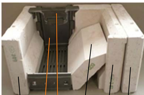
Modell 624 und 634 / Türbandung rechts (Feuer links)
